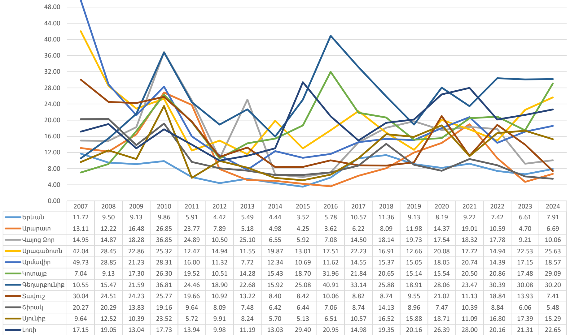
Մեկ սպառողին բաժին ընկնող էլեկտրամատակարարման ընդհատումների միջին տարեկան տևողությունը Հայաստանի Հանրապետության մարզերում և Երևան քաղաքում 2007-2024թթ. (SAIDI, ժամ/սպառող)
