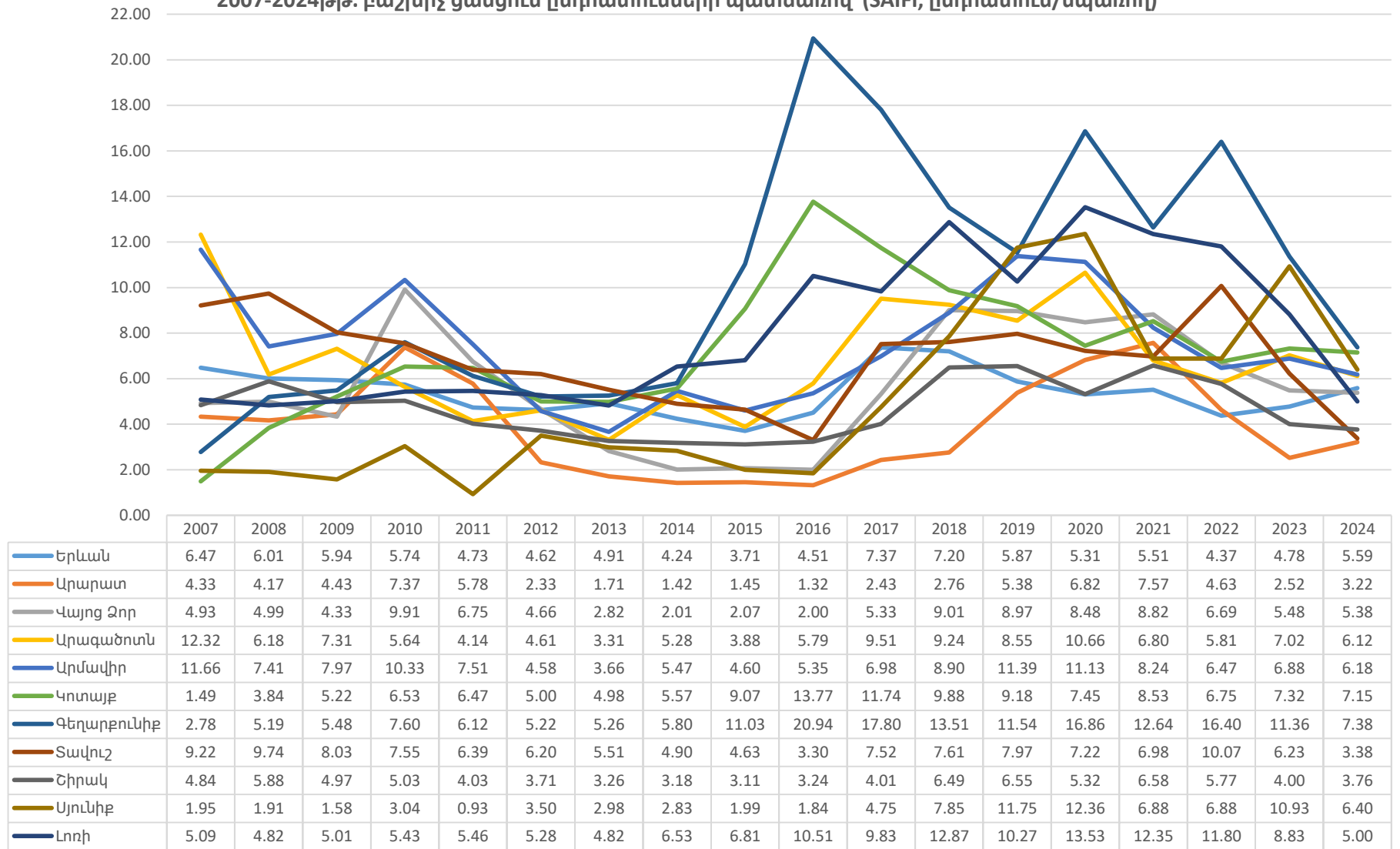
Մեկ սպառողին բաժին ընկնող էլեկտրամատակարարման ընդհատումների միջին տարեկան քանակությունը Հայաստանի Հանրապետության մարզերում և Երևան քաղաքում 2007-2024թթ. բաշխիչ ցանցում ընդհատումների պատճառով (SAIFI, ընդհատում/սպառող)
