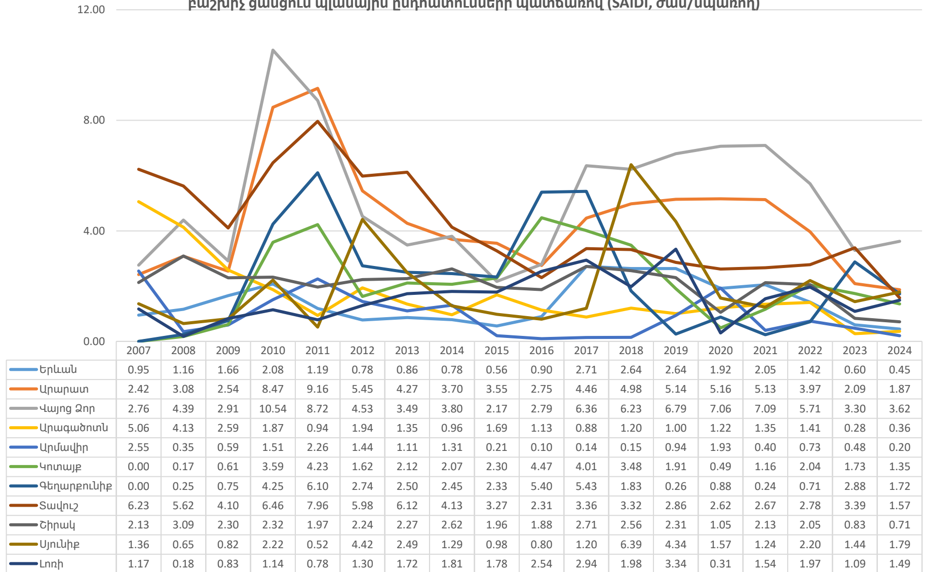
Մեկ սպառողին բաժին ընկնող էլեկտրամատակարարման ընդհատումների միջին տարեկան տևողությունը Հայաստանի Հանրապետությունում 2007-2024թթ. բաշխիչ ցանցում պլանային ընդհատումների պատճառով (SAIDI, ժամ/սպառող)
