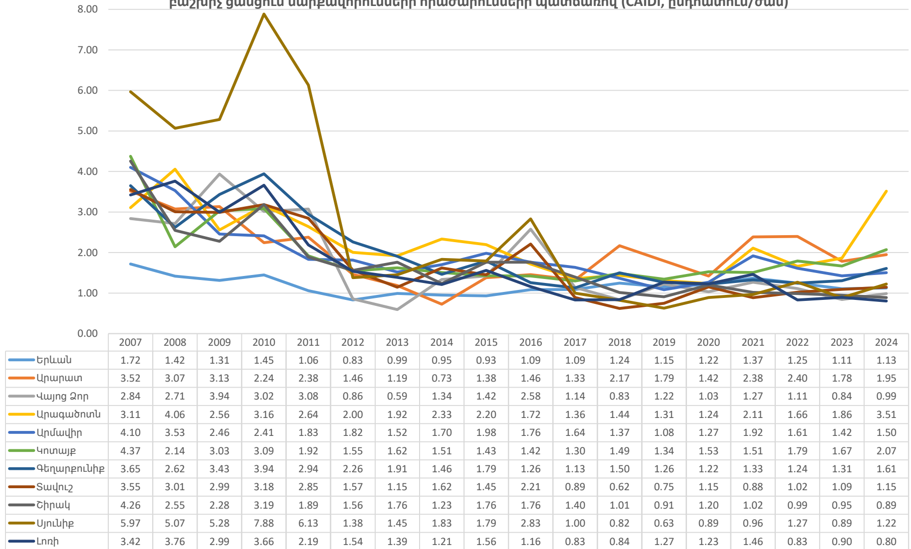
Էլեկտրամատակարարման ընդհատումների վերականգնման միջին տարեկան տևողությունը Հայաստանի Հանրապետությունում 2007-2024թթ. բաշխիչ ցանցում սարքավորումների հրաժարումների պատճառով (CAIDI, ընդհատում/ժամ)
