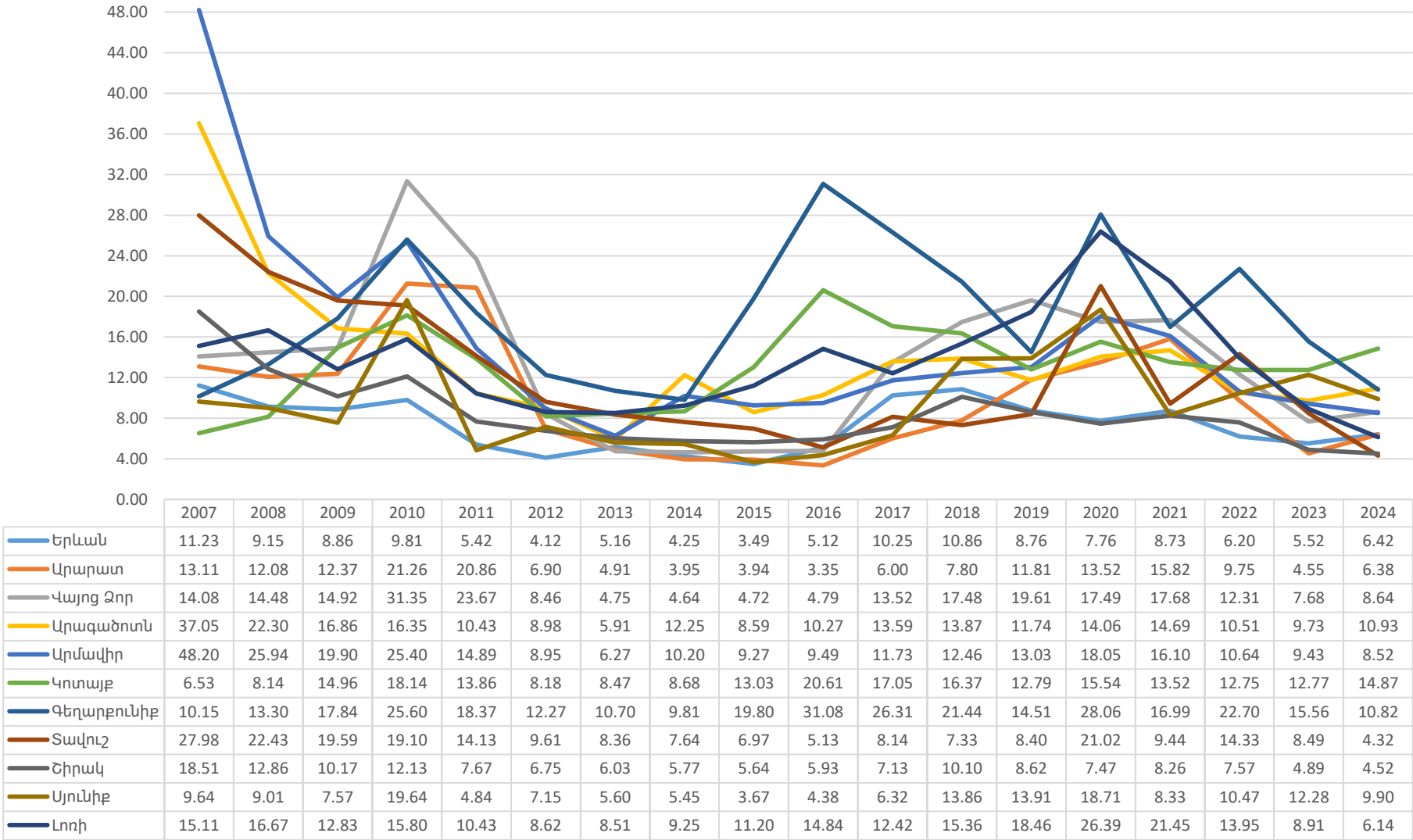
Մեկ սպառողին բաժին ընկնող էլեկտրամատակարարման ընդհատումների միջին տարեկան տևողությունը Հայաստանի Հանրապետության մարզերում և Երևան քաղաքում 2007-2024թթ. բաշխիչ ցանցում ընդհատումների պատճառով (SAIDI, ժամ/սպառող)
