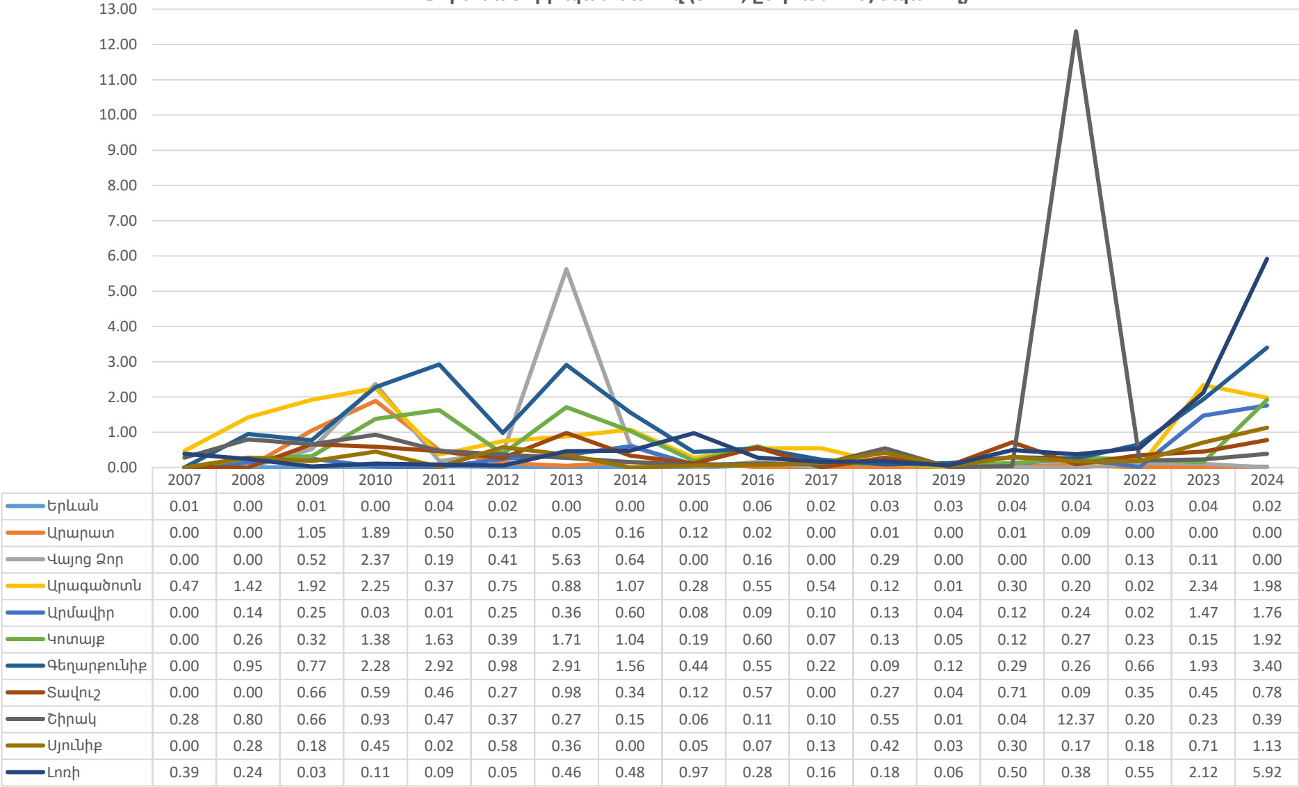
Մեկ սպառողին բաժին ընկնող էլեկտրամատակարարման ընդհատումների միջին տարեկան քանակությունը Հայաստանի Հանրապետությունում 2007-2024թթ. Ֆորս-մաժորի պատճառով (SAIFI, ընդհատում/սպառող)
