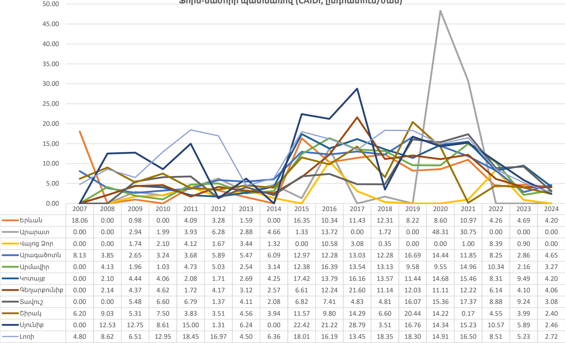
Էլեկտրամատակարարման ընդհատումների վերականգնման միջին տարեկան տևողությունը Հայաստանի Հանրապետությունում 2007-2024թթ. Ֆորս-մաժորի պատճառով (CAIDI, ընդհատում/ժամ)
