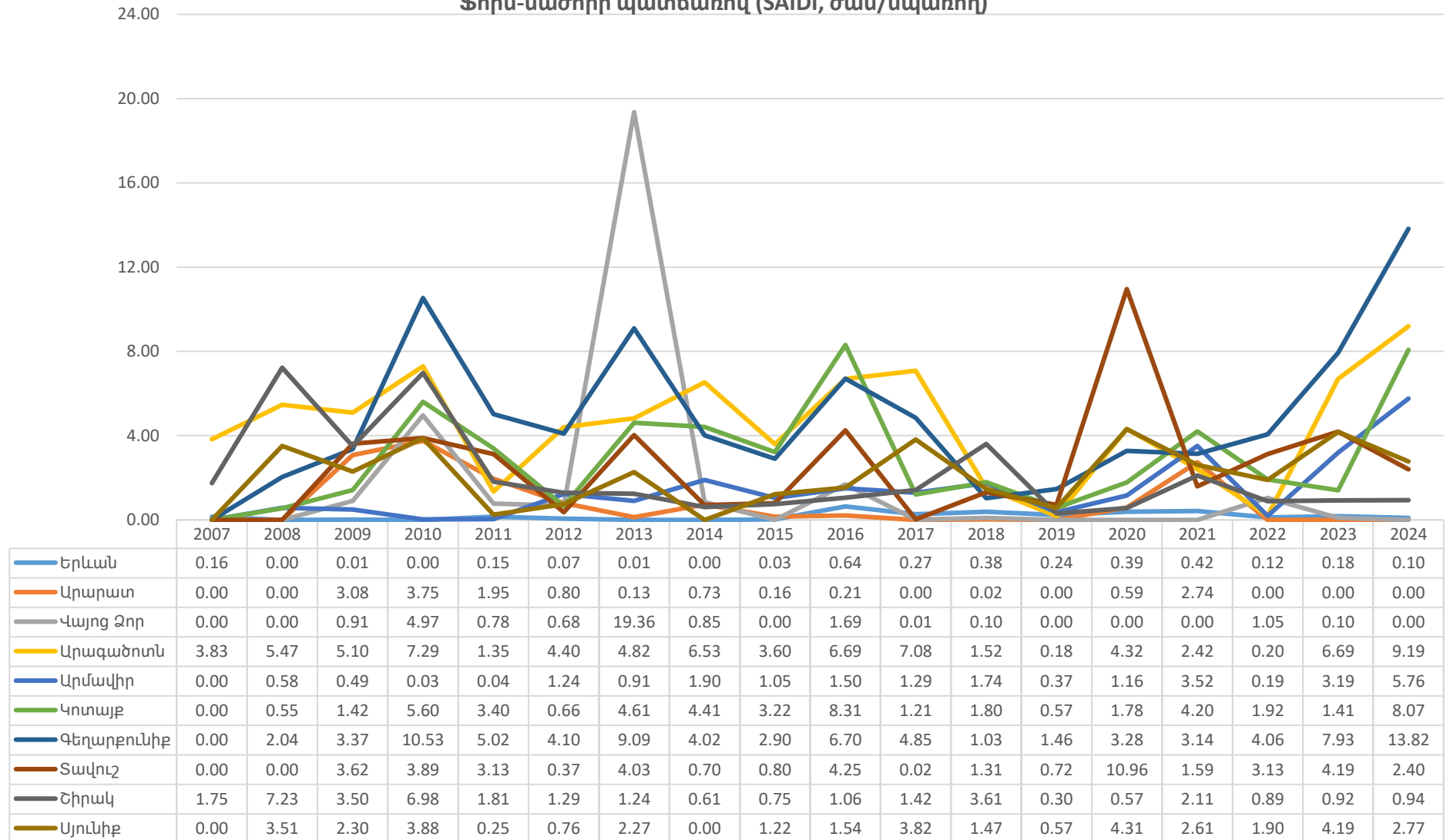
Մեկ սպառողին բաժին ընկնող էլեկտրամատակարարման ընդհատումների միջին տարեկան տևողությունը Հայաստանի Հանրապետությունում 2007-2024թթ. Ֆորս-մաժորի պատճառով (SAIDI, ժամ/սպառող)
