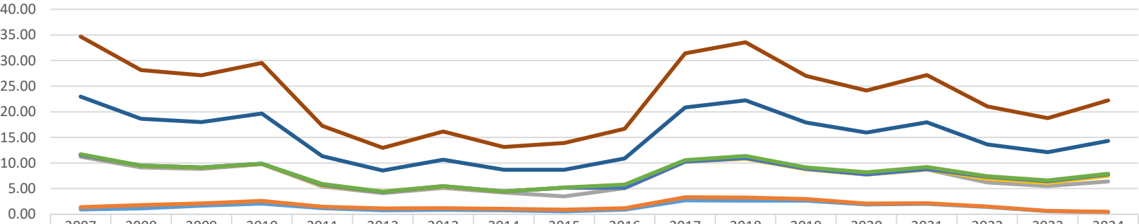
Մեկ սպառողին բաժին ընկնող էլեկտրամատակարարման ընդհատումների միջին տարեկան տևողությունը Երևան քաղաքում 2007-2024թթ. (SAIDI, ժամ/սպառող)
