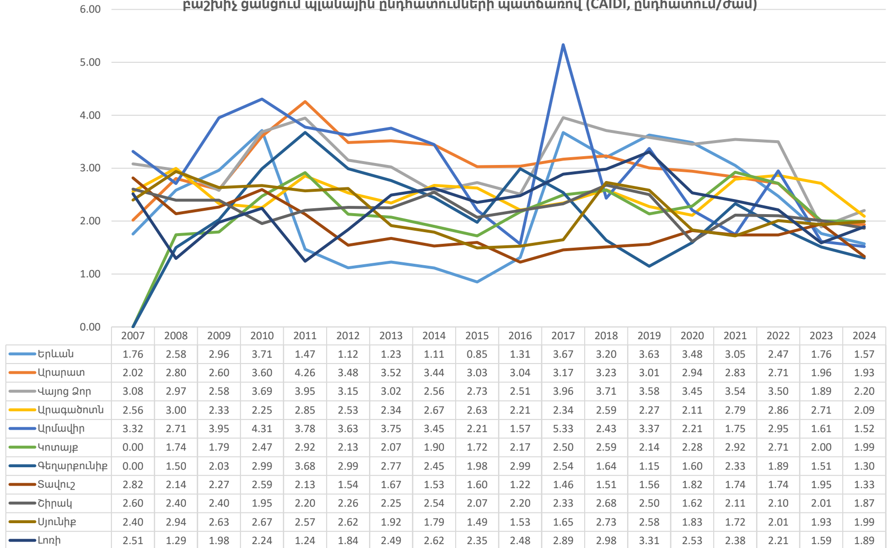
Էլեկտրամատակարարման ընդհատումների վերականգնման միջին տարեկան տևողությունը Հայաստանի Հանրապետությունում 2007-2024թթ. բաշխիչ ցանցում պլանային ընդհատումների պատճառով (CAIDI, ընդհատում/ժամ)
