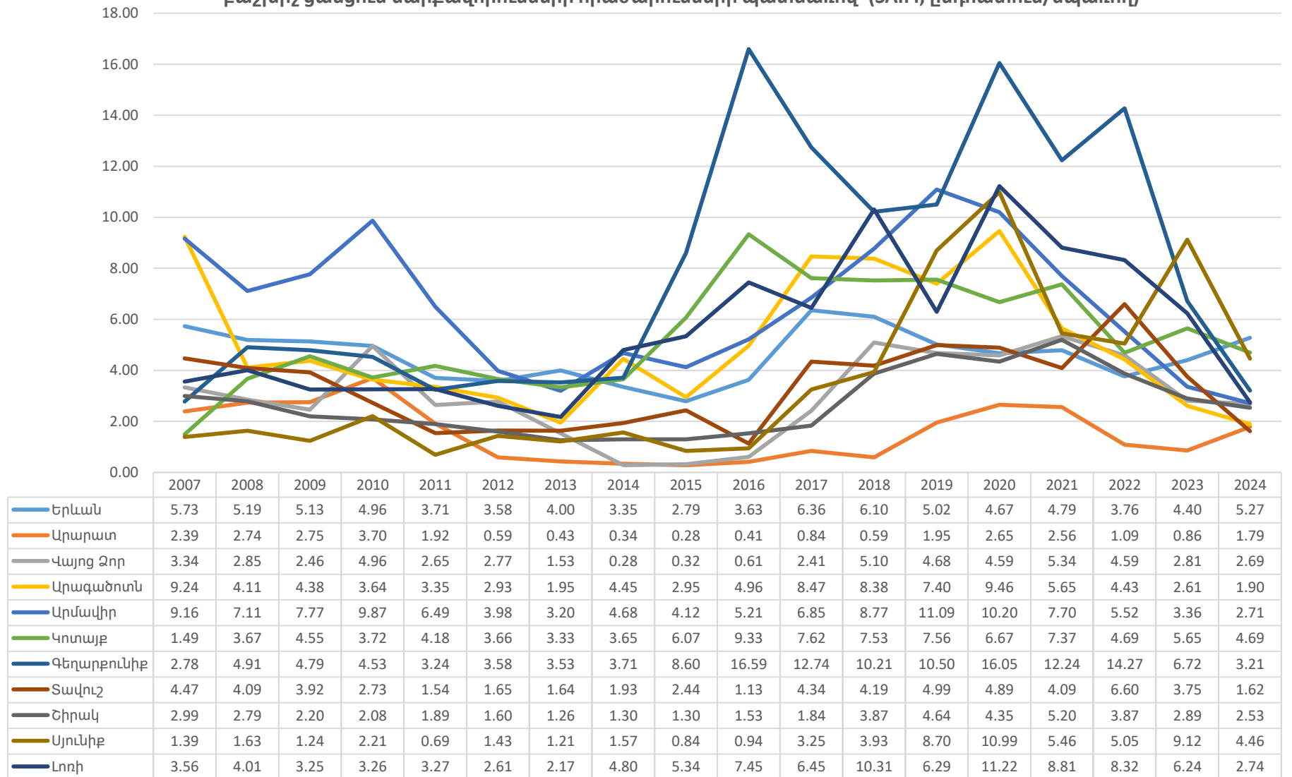
Մեկ սպառողին բաժին ընկնող էլեկտրամատակարարման ընդհատումների միջին տարեկան քանակությունը Հայաստանի Հանրապետությունում 2007-2024թթ. բաշխիչ ցանցում սարքավորումների հրաժարումների պատճառով (SAIFI, ընդհատում/սպառող)
