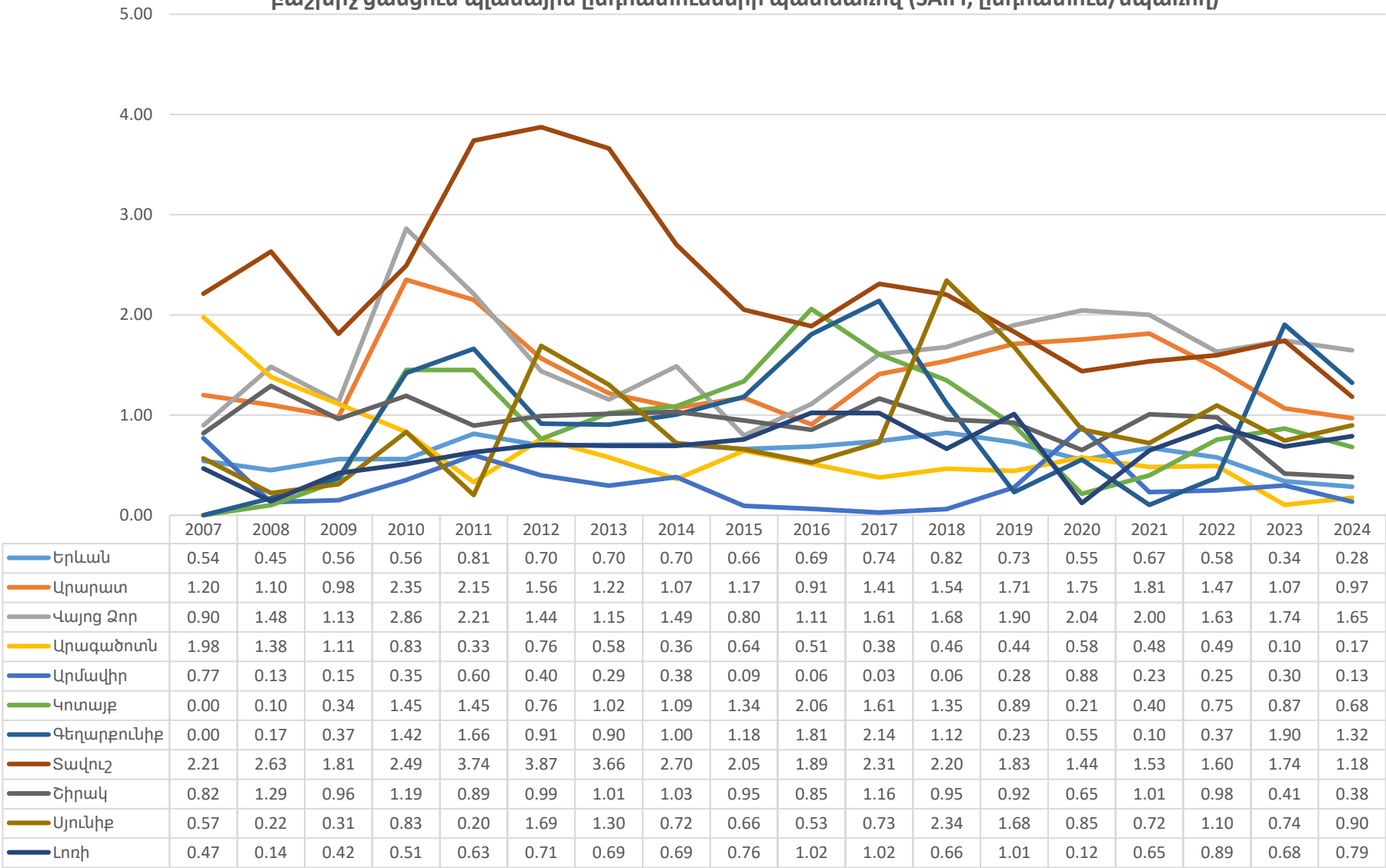
Մեկ սպառողին բաժին ընկնող էլեկտրամատակարարման ընդհատումների միջին տարեկան քանակությունը Հայաստանի Հանրապետությունում 2007-2024 թթ. բաշխիչ ցանցում պլանային ընդհատումների պատճառով (SAIFI, ընդհատում/սպառող)
