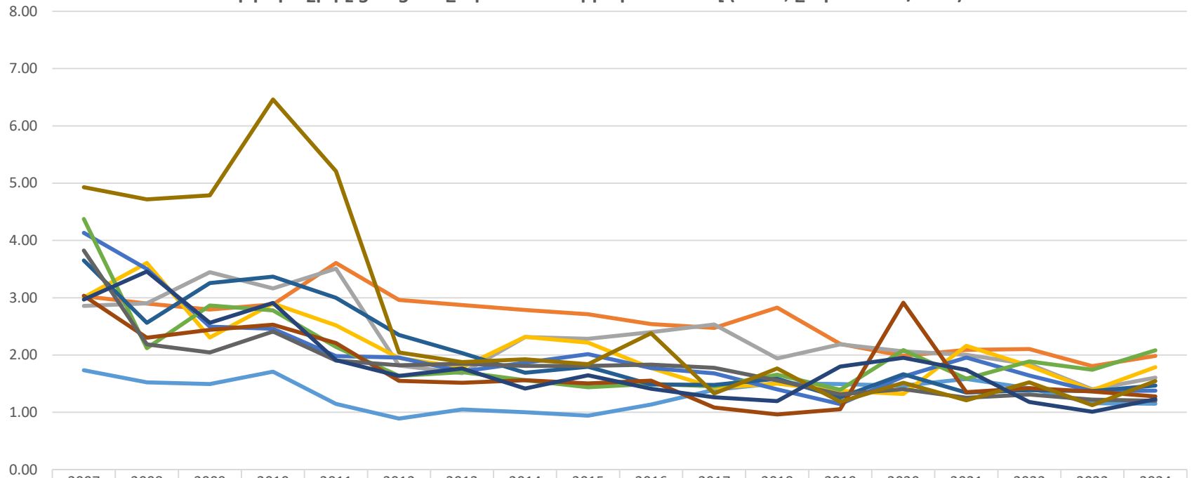
Էլեկտրամատակարարման ընդհատումների վերականգնման միջին տարեկան տևողությունը Հայաստանի Հանրապետության մարզերում և Երևան քաղաքում 2007-2024թթ. բաշխիչ ցանցում ընդհատումների պատճառով (CAIDI, ընդհատում/ժամ)
