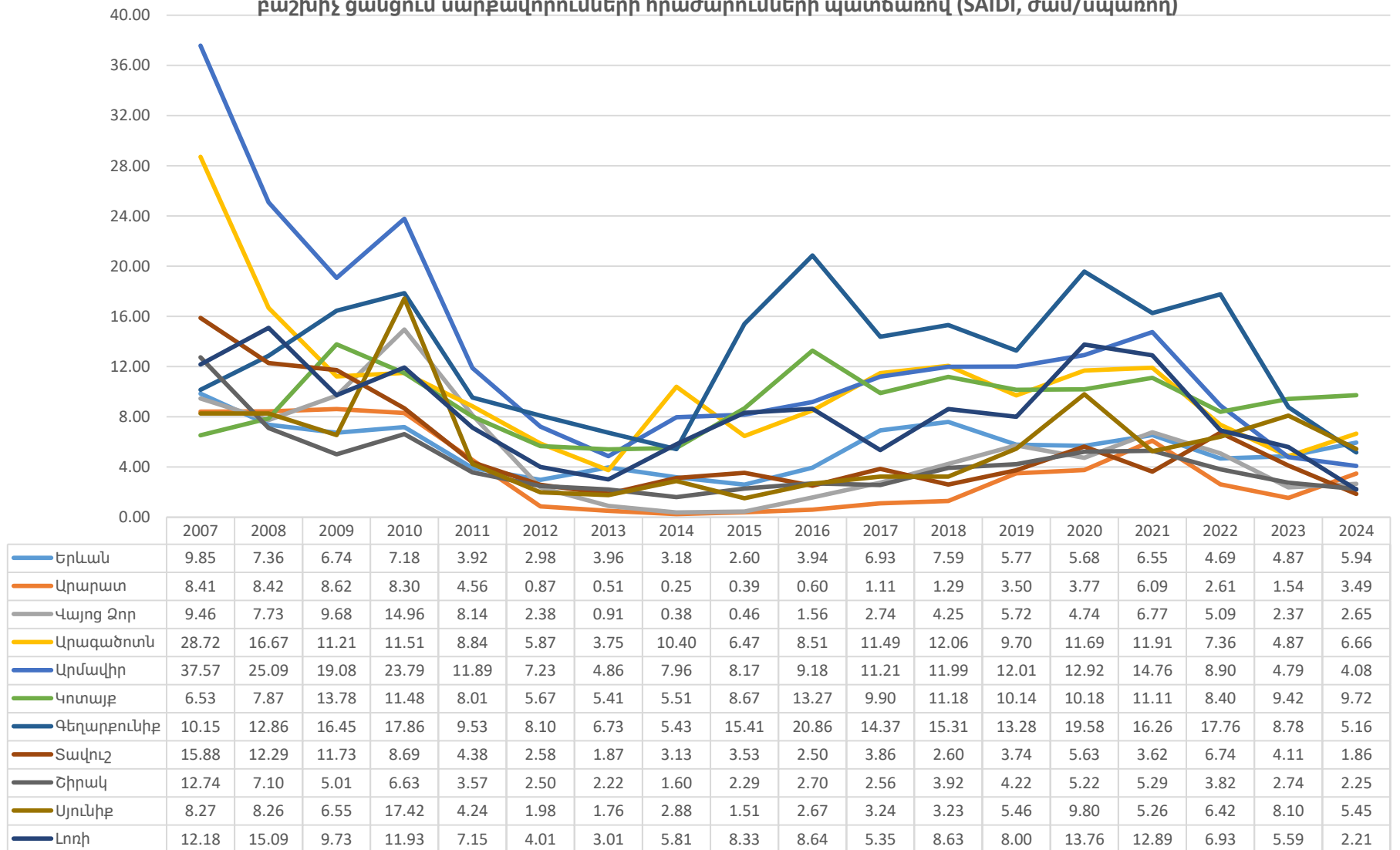
Մեկ սպառողին բաժին ընկնող էլեկտրամատակարարման ընդհատումների միջին տարեկան տևողությունը Հայաստանի Հանրապետությունում 2007-2024թթ. բաշխիչ ցանցում սարքավորումների հրաժարումների պատճառով (SAIDI, ժամ/սպառող)
