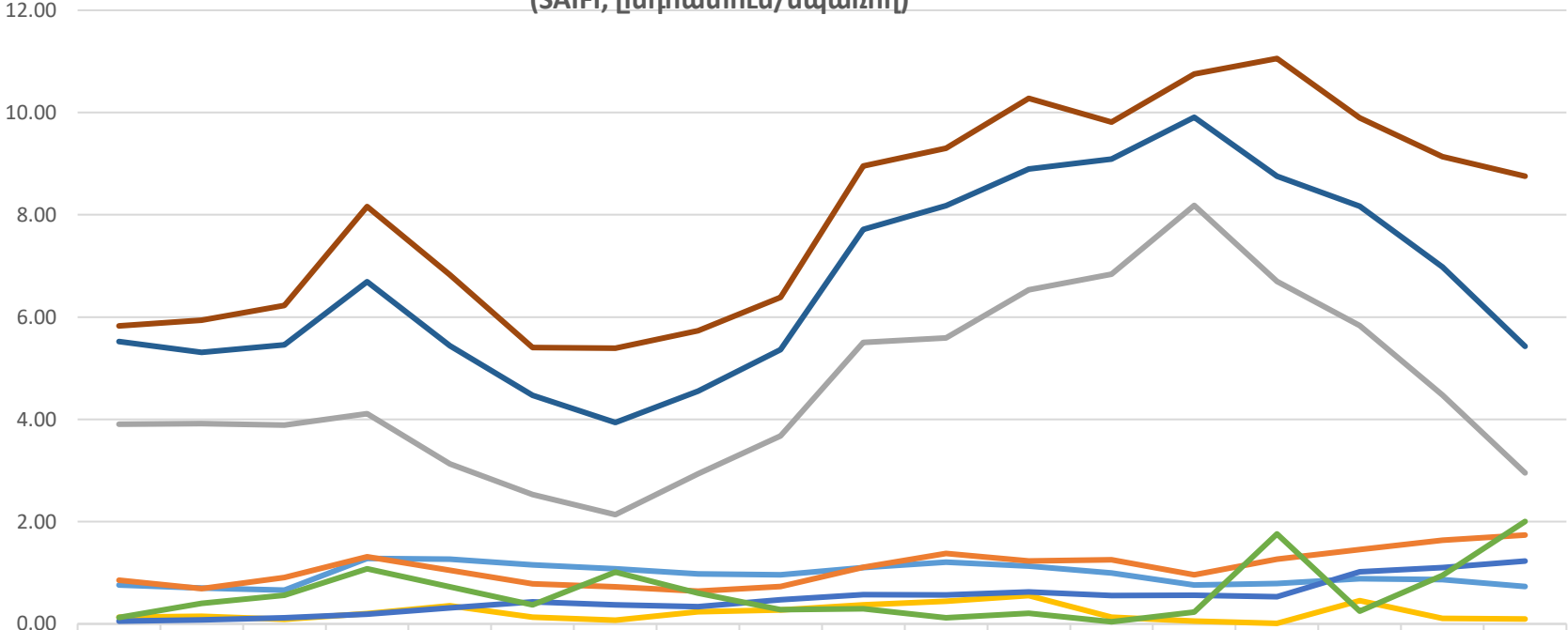
Մեկ սպառողին բաժին ընկնող էլեկտրամատակարարման ընդհատումների միջին տարեկան քանակությունը Հայաստանի Հանրապետության մարզերում 2007-2024թթ. (SAIFI, ընդհատում/սպառող)
