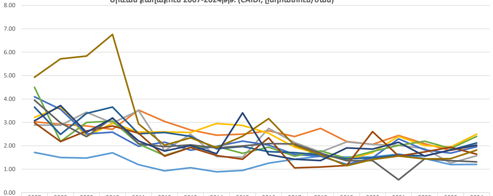
Էլեկտրամատակարարման ընդհատումների վերականգնման միջին տարեկան տևողությունը Հայաստանի Հանրապետության մարզերում և Երևան քաղաքում 2007-2024թթ. (CAIDI, ընդհատում/ժամ)
