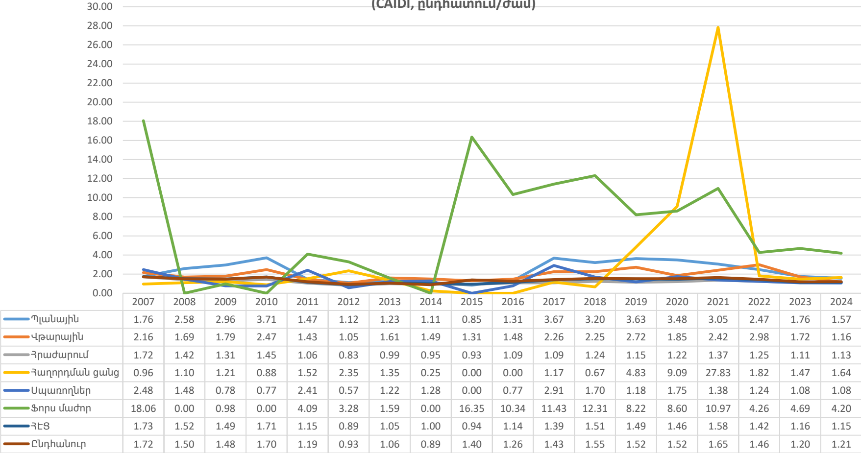
Էլեկտրամատակարարման ընդհատումների վերականգնման միջին տարեկան տևողությունը Երևան քաղաքում 2007-2024թթ. (CAIDI, ընդհատում/ժամ)
